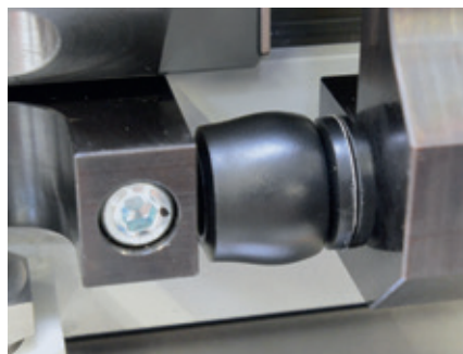
主轴尾座活动轴内的急停保护
