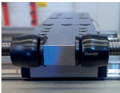
直线电缸生产模块内的终端位置缓冲装置
