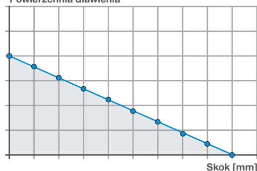
Powierzchnia dławienia
