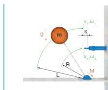
R4.在传动力矩作用下向上摆动的物体 a) 水平碰撞时
