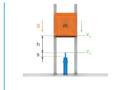
L2.在反作用传动力作用下向下运动的物体
