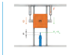
L4.在传动力作用下向上运动的物体
