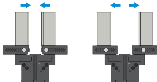
조정 가능한 조 - EB5000 공구 없이 그리핑 범위를 조정하기 위한 용도
