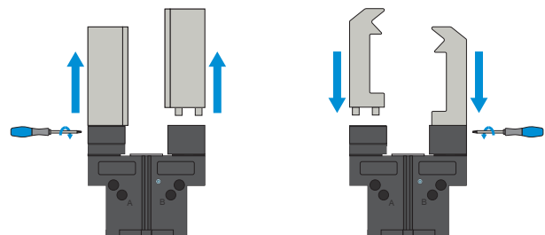
교체 가능한 조 - WB5000 맞춤형 그리퍼 핑거의 신속한 교체 가능
