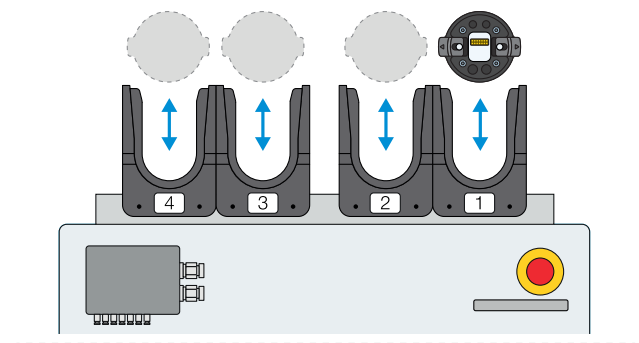
Mit der Ablagestation für bis zu vier MATCH-Komponenten kann die Flexibilität bis auf das Höchste gesteigert werden
