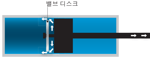
댐퍼 리턴
