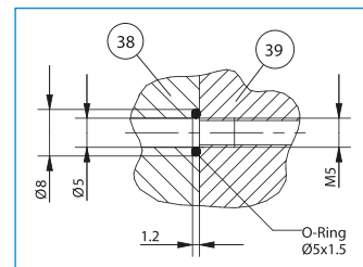
Tomada de aire directa sin tubos
