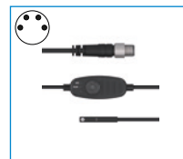
MFS02-S-KHC-IL 直式位置传感器, 电缆 0.3 米 - 插头 M8
