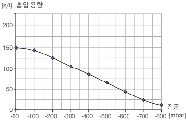
다양한 진공 레벨에서의 흡입 용량
