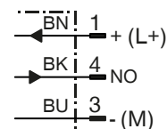
Schemat przyłączeniowy
