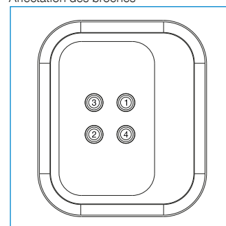
Affectation des broches
