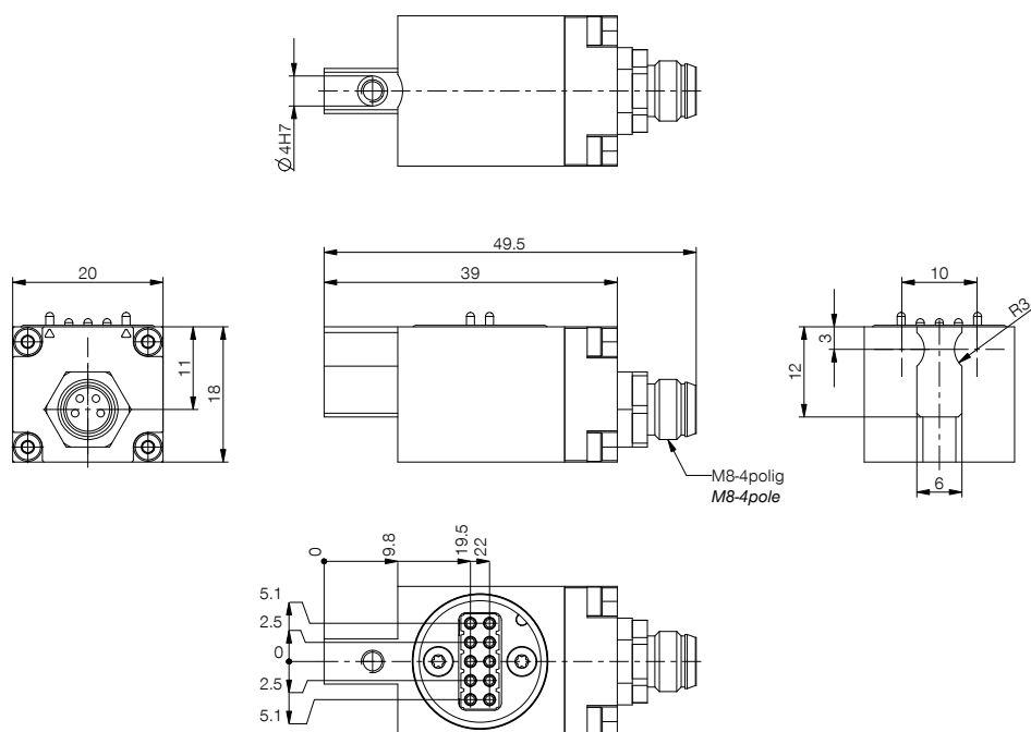
PIN - Belegung
