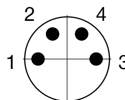
Disposición de los pines
