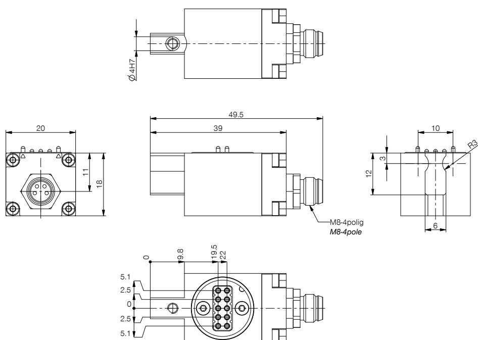
Obłożenie PIN-ów
