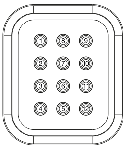
Obłożenie PIN-ów
