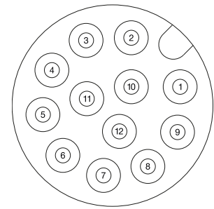
Obłożenie PIN-ów
