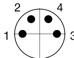
Obłożenie PIN-ów
