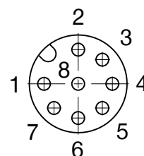
PIN - Belegung
