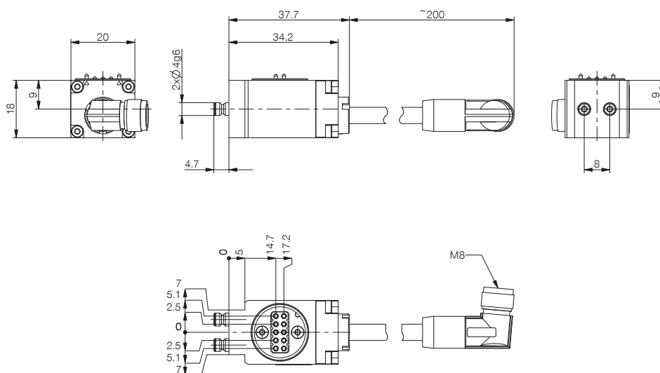
PIN - Belegung
