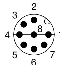
Obłożenie PIN-ów
