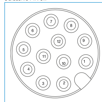
Obłożenie PIN-ów
