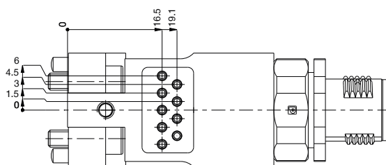
PIN - Belegung
