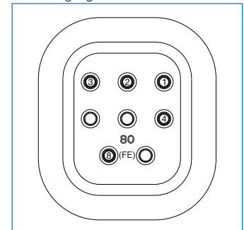
PIN - Belegung
