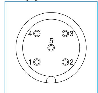
PIN - Belegung
