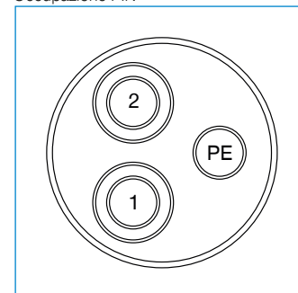
Occupazione PIN
