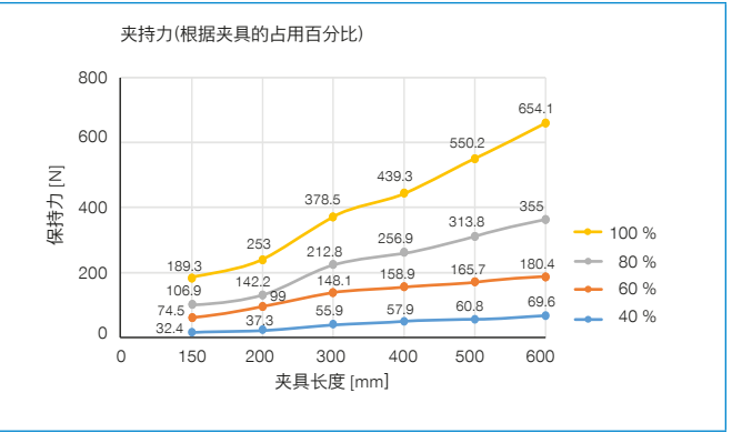
ZGM40 椭圆形
