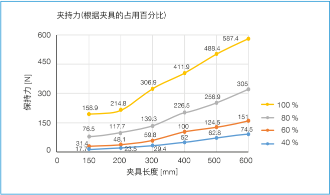
ZGM40 圆形
