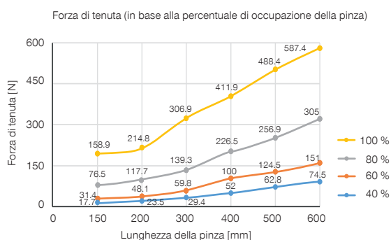
ZGM40 rotondo
