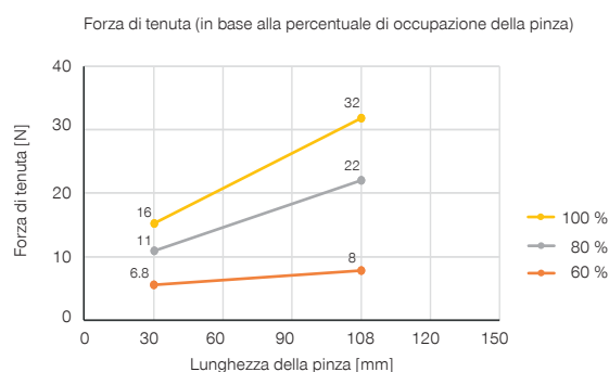
ZGM20 rotondo
