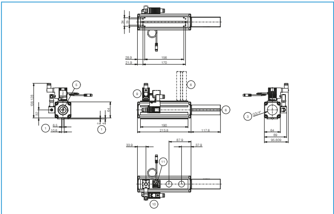
ZMP30303-A-AR3-DL-SN / -SP
