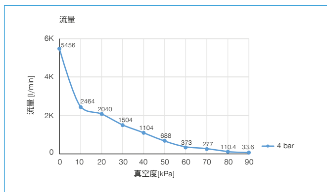
ZMP30316
