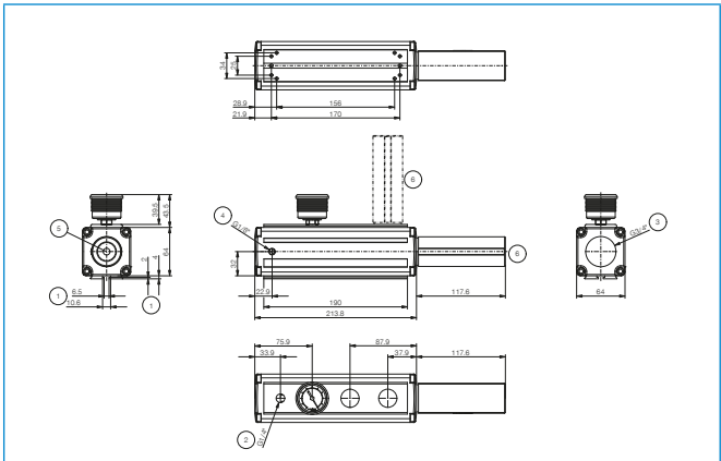
ZMP30303
