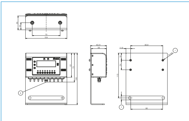
① Upevnenie
