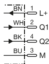
Anschlussplan
