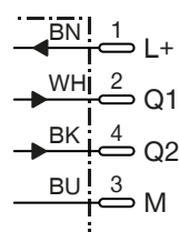
Schemat przyłączeniowy
