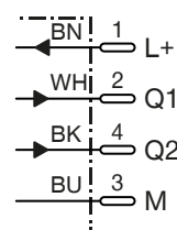
Esquema de conexiones
