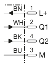
Esquema de conexiones
