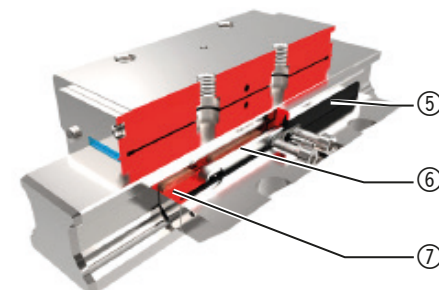
Abb. 2: Element KBH im Schnitt
